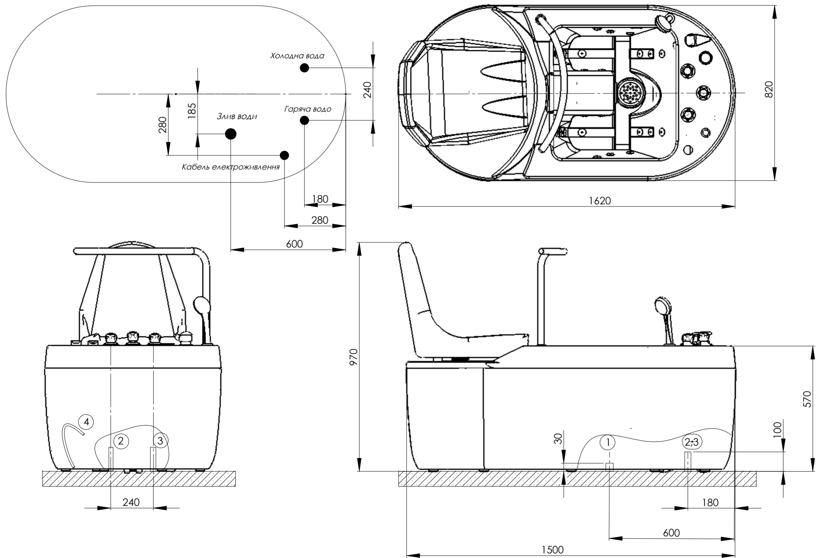
Схема підведення комунікацій до ванни AQUASMART
